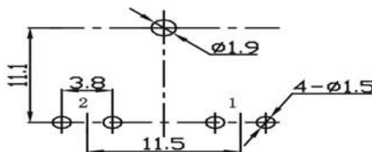
印制板开孔尺寸(±0.1mm)
